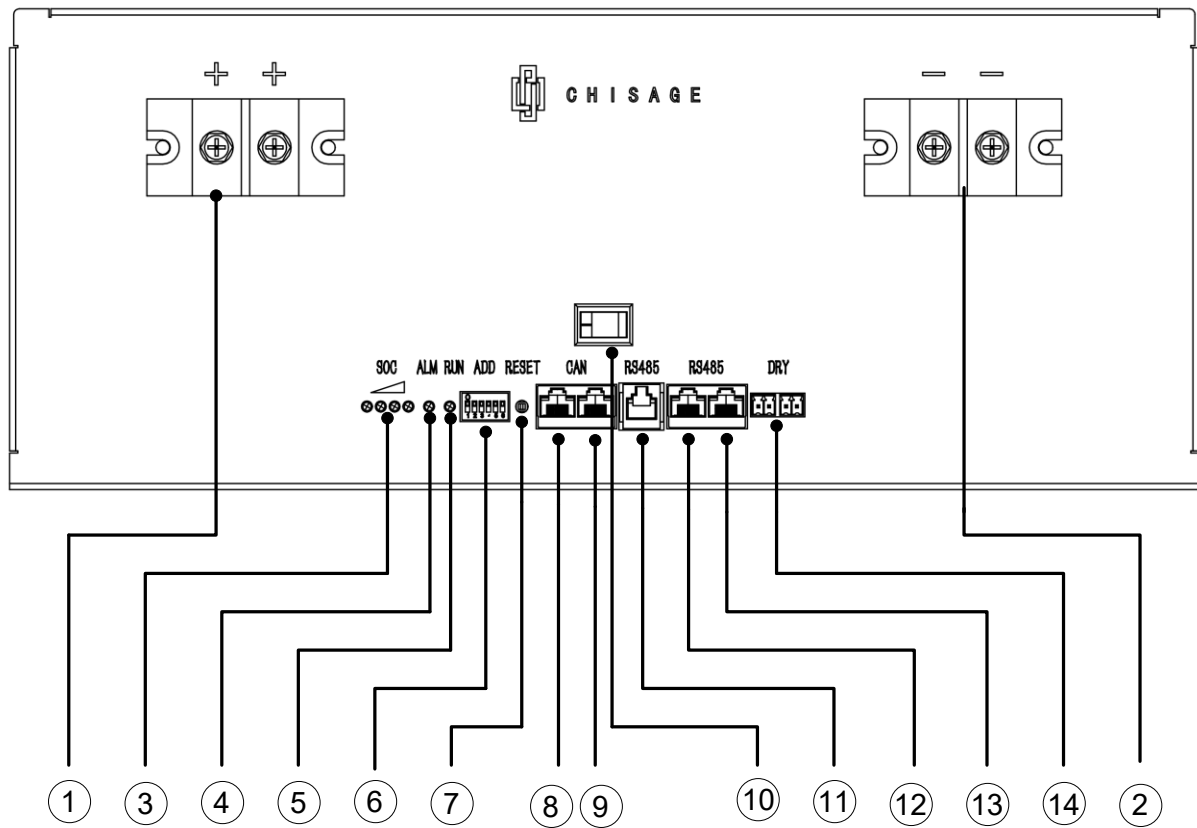
Fig. 3-5 CE48100-R PACK interface
