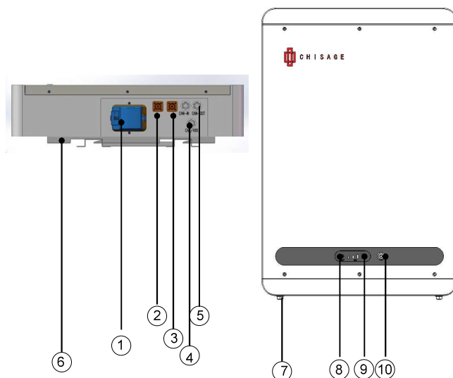
Fig. 3-5 CE48100-W PACK interface
